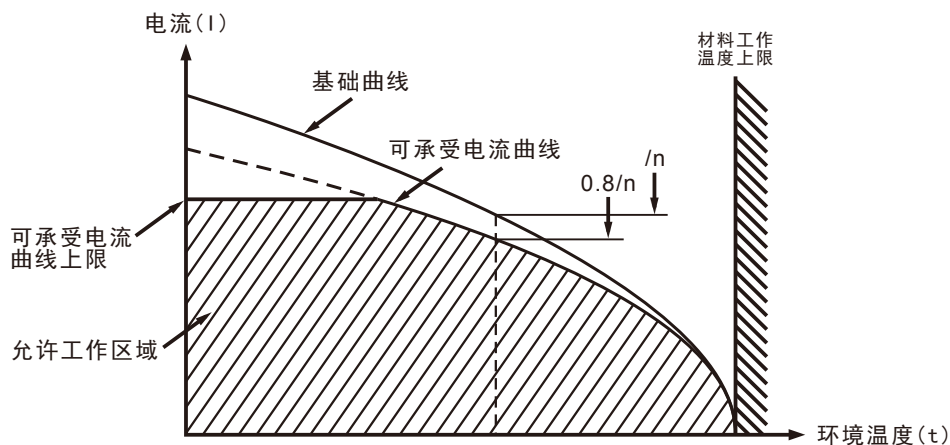
电流载流能力曲线图
